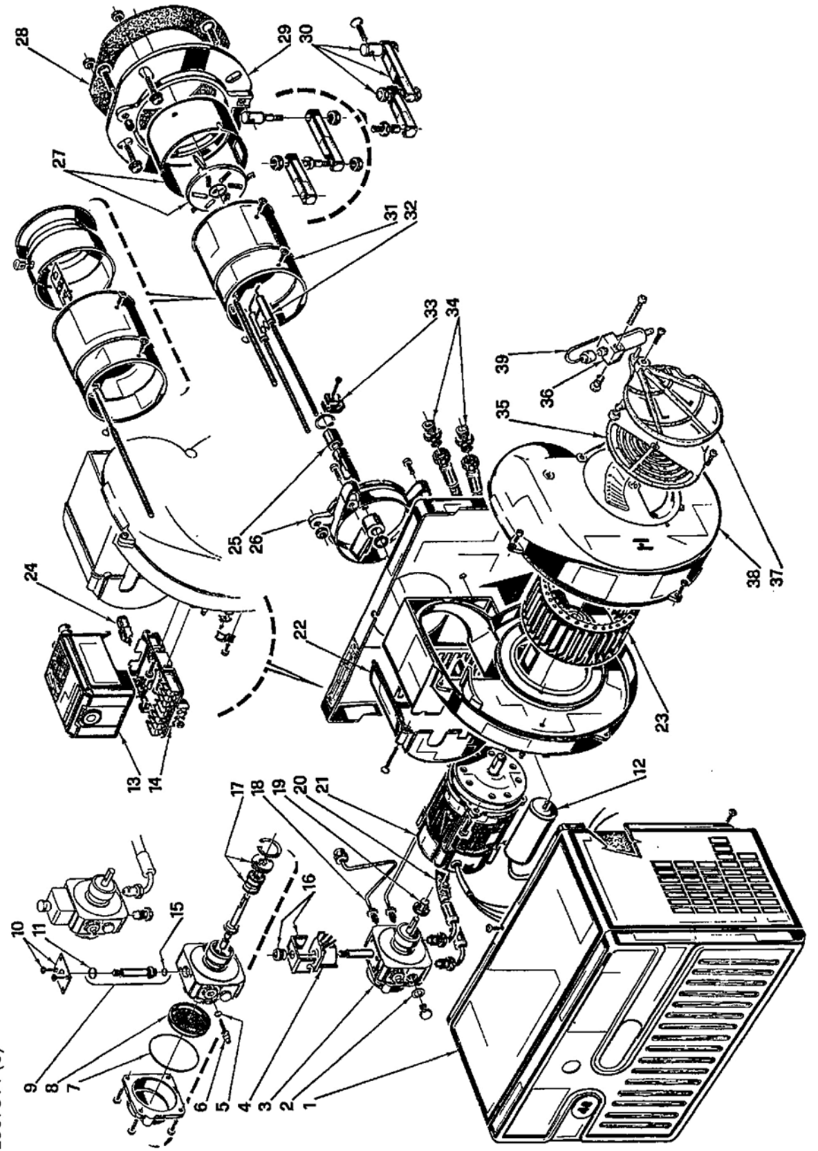
G20 油バーナ 部品図
