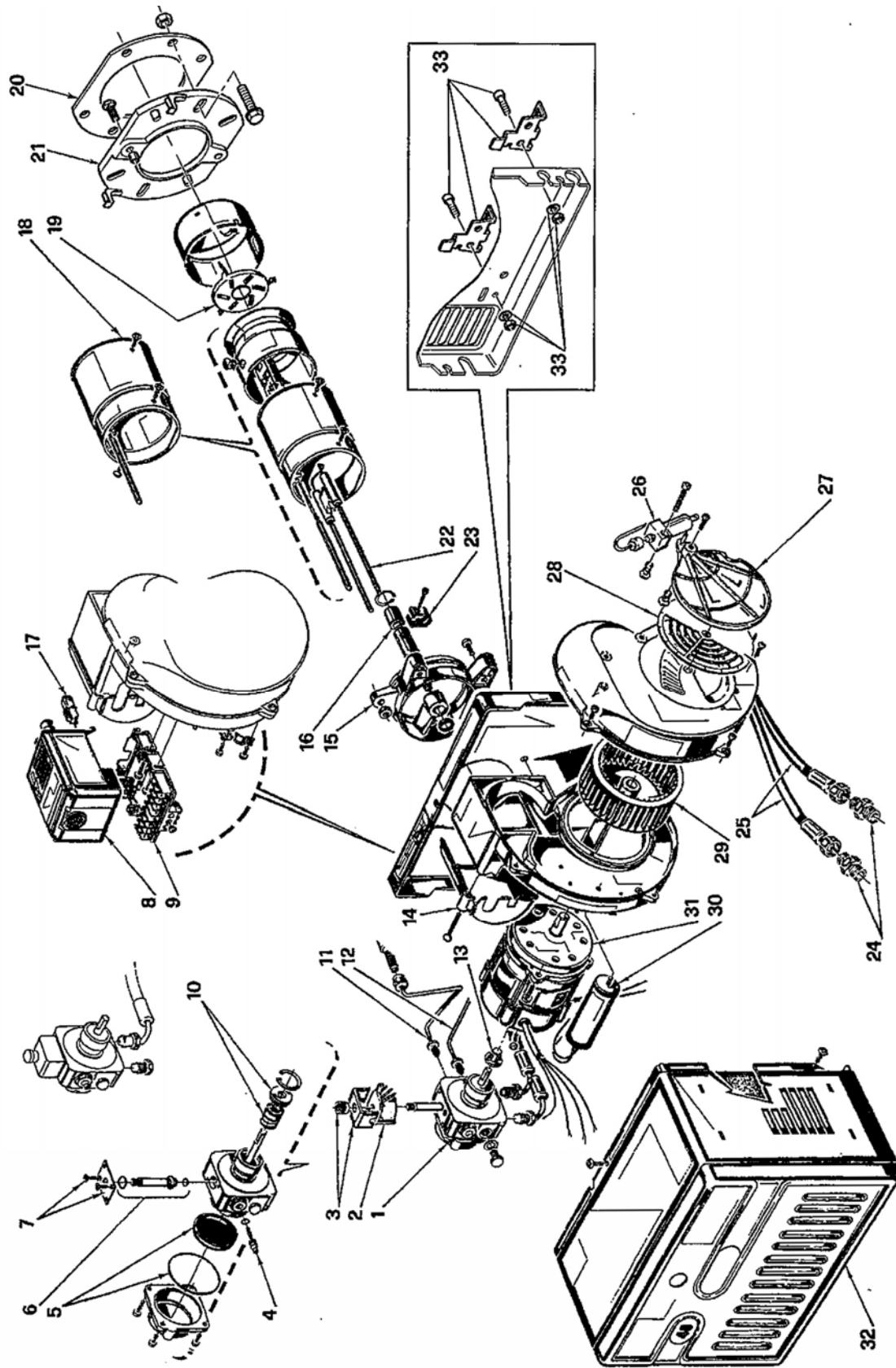
G10 油バーナ 部品図
